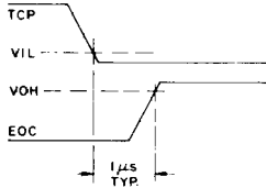
Fig.17 EOC TURN-ON
