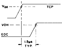
Fig.39 EOC TURN-ON
