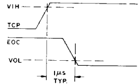
Fig.19 EOC TURN-OFF
